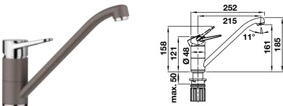
Auslauf 180° schwenkbar
