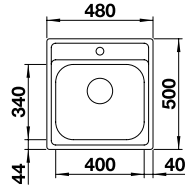
Ausschnitt: 462 x 482 mm Beckentiefe: 158 mm Außenmaß: 480 x 500 mm Mindesteinbauhöhe: 283 mm
