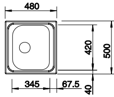
Ausschnitt: 462 x 482 mm Beckentiefe: 160 mm Außenmaß: 480 x 500 mm Mindesteinbauhöhe: 300 mm
