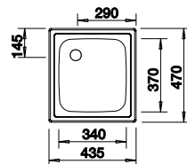
Ausschnitt: 417 x 452 mm Beckentiefe 150 mm Außenmaß 435 x 470 mm Mindesteinbauhöhe: 285 mm
