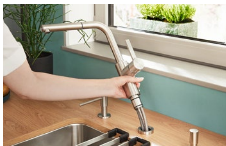
herausnehmbare Vorfenster-Armatur (zur Seite/ins Becken legen)
